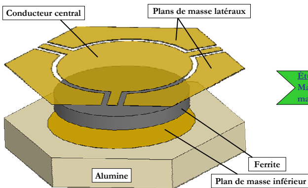
Circulateur coplanaire
